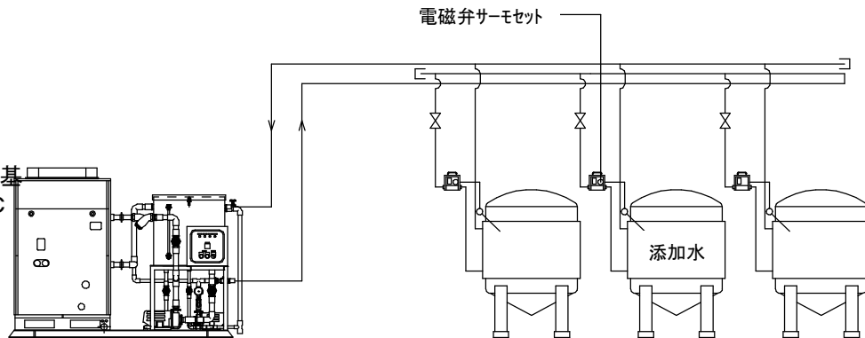
FRU-N1002ALVK-S
