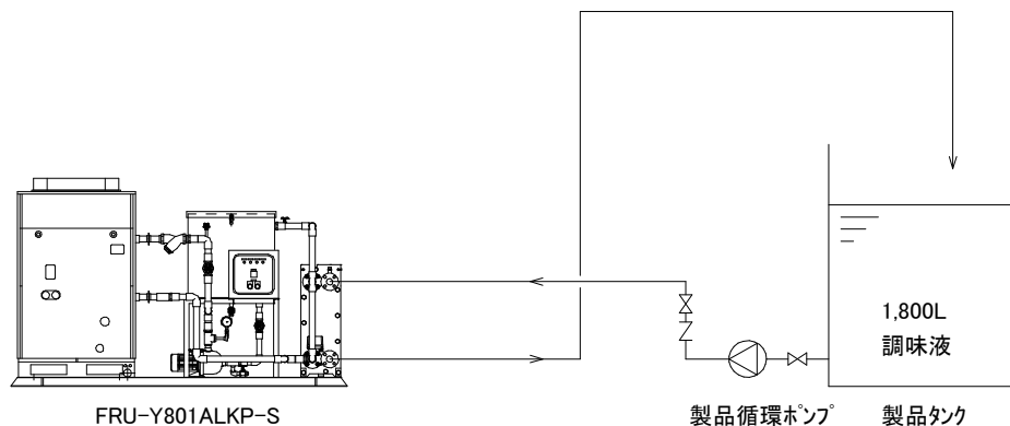
FRU-Y801ALKP-S
